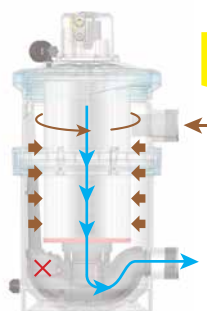
Wasserfluss im Filterbetrieb
